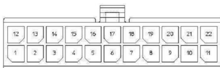
22-CKT.
