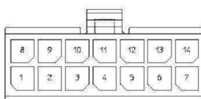
14-CKT.
