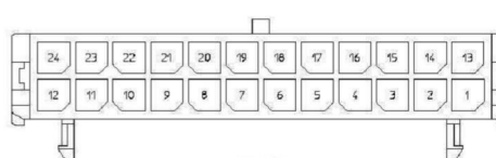
24-CKT.
