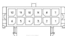
12-CKT.
