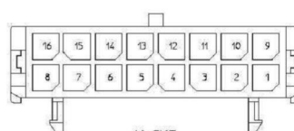
16-CKT.
