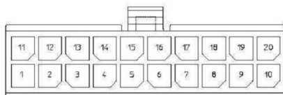
20-CKT.
