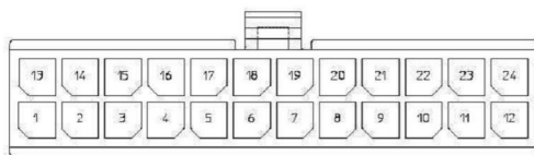
24-CKT.
