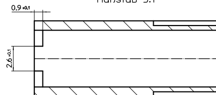
Schnitt B-B Maßstab 5:1
