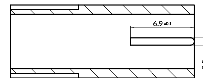
Schnitt C-C Maßstab 5:1
