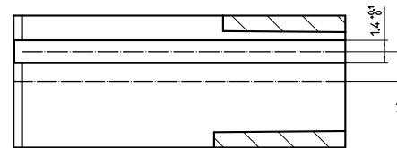
Schnitt A-A Maßstab 5:1
