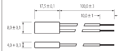
Maßzeichnung P8
