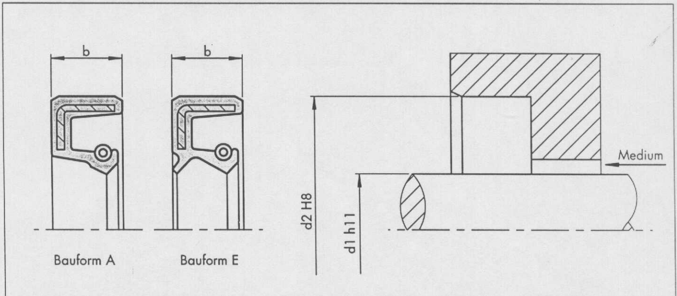
Bild 18 Einbauzeichnung
