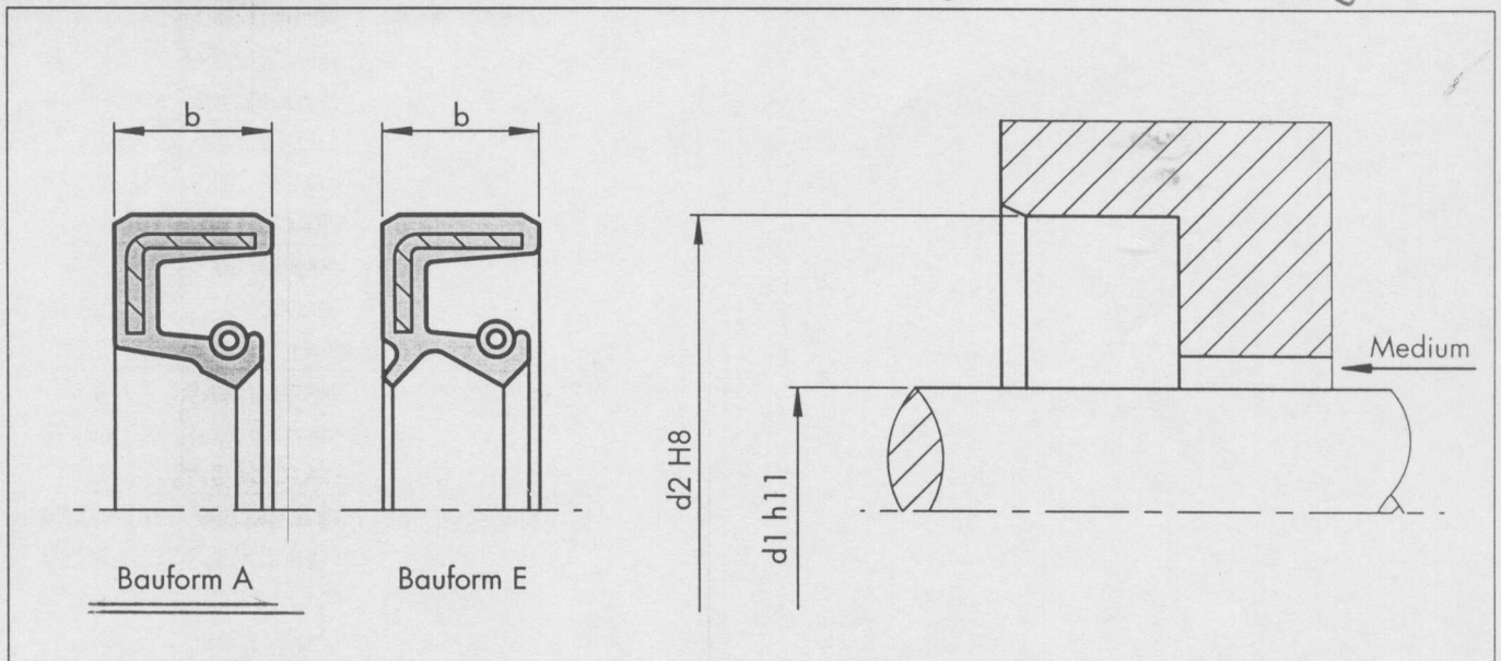
Bild 18 Einbauzeichnung
