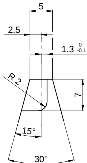
DETTAGLIO A 2:1
