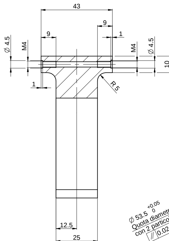
SEZIONE A-A
