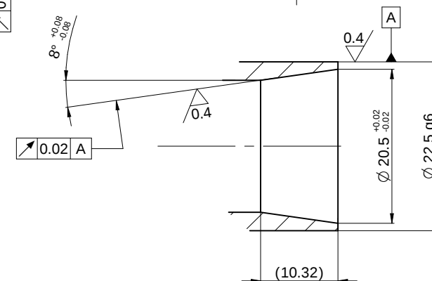
DETTAGLIO B
