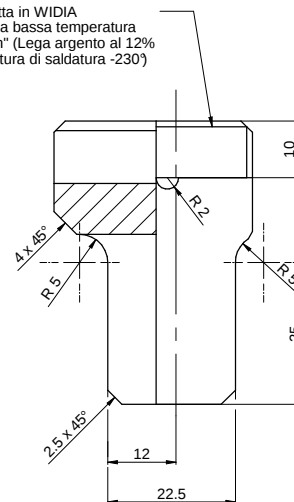
SEZIONE A-A
