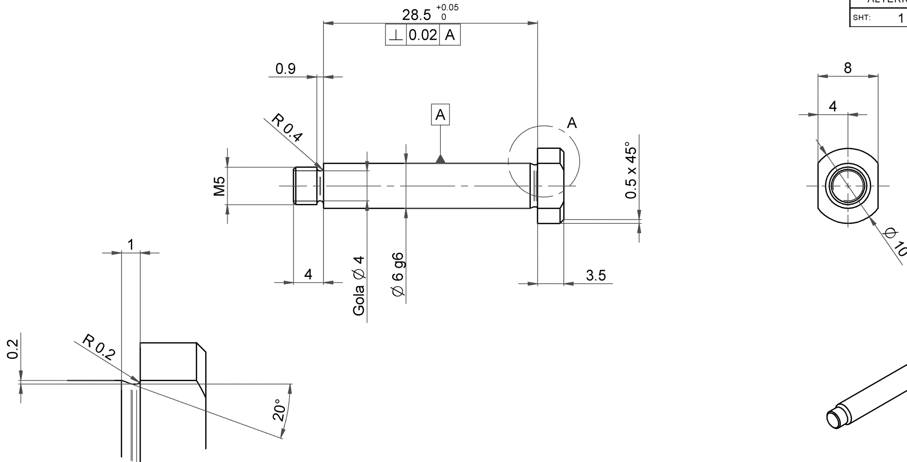
DETTAGLIO A 5:1
