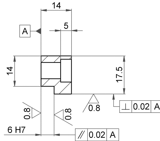
SEZIONE A-A
