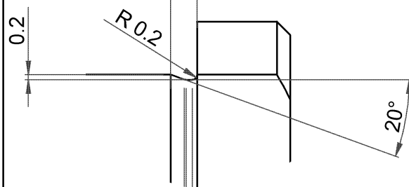
DETTAGLIO A 5:1
