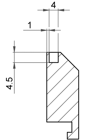
SEZIONE A-A
