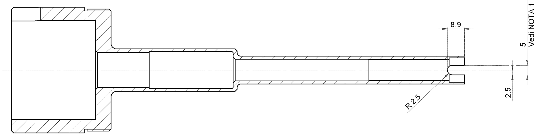
SEZIONE A-A
