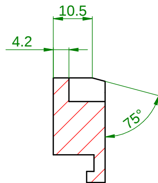
SEZIONE B-B
