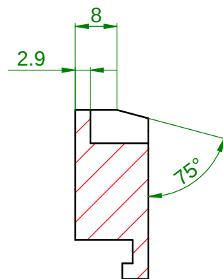
SEZIONE B-B
