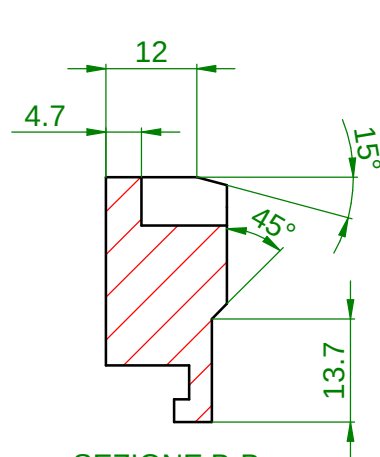
SEZIONE B-B
