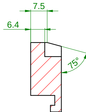
SEZIONE B-B
