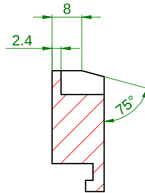
SEZIONE B-B
