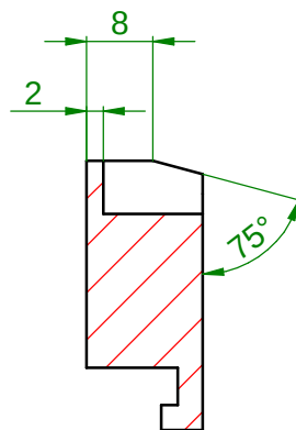
SEZIONE B-B
