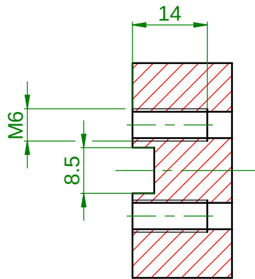
SEZIONE B-B
