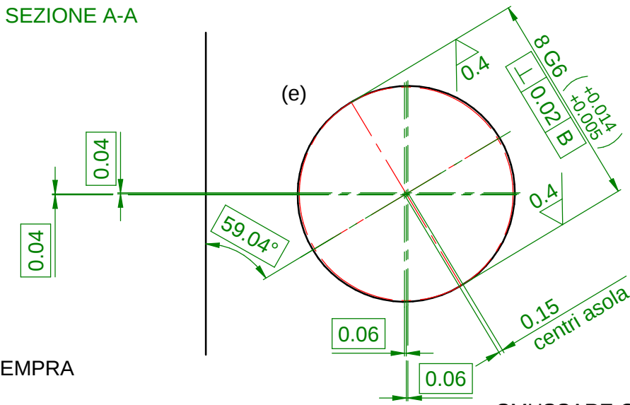
DETTAGLIO C
