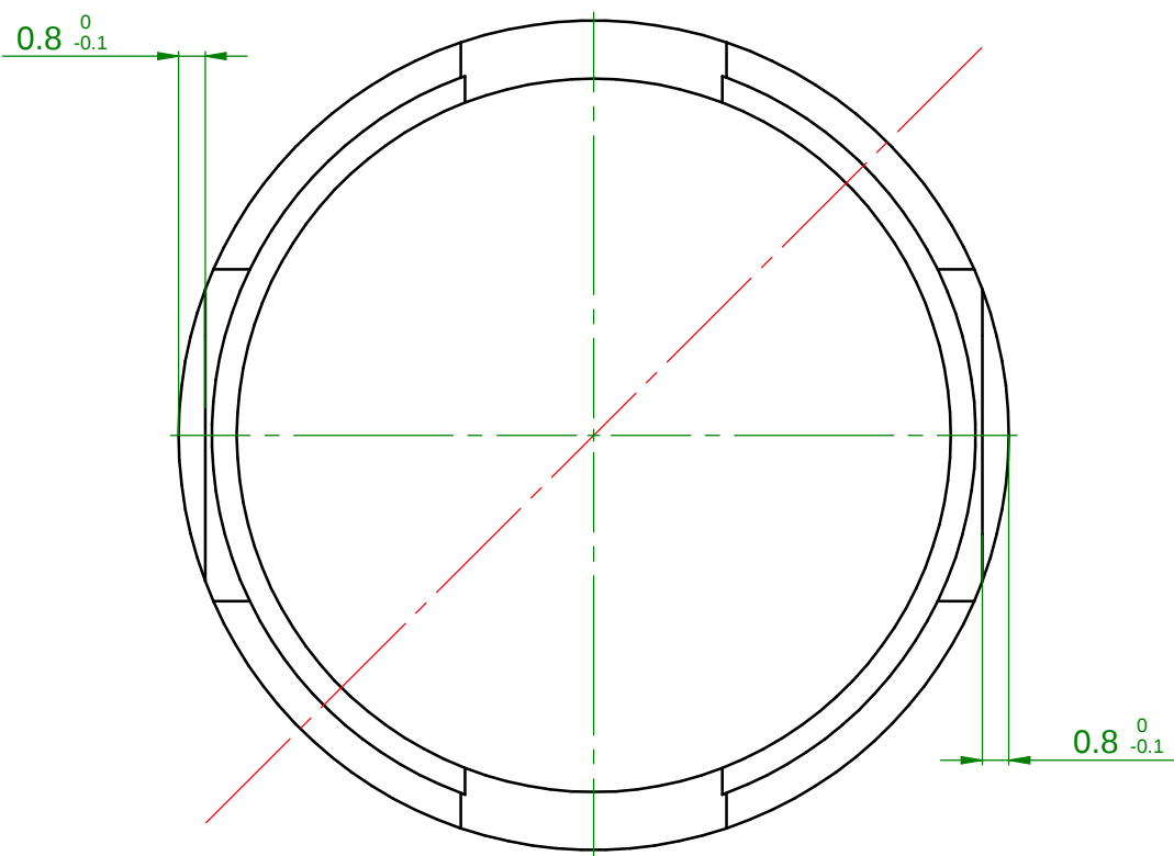
DETTAGLIO C
