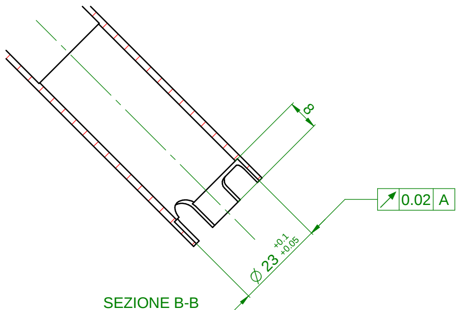
SEZIONE B-B
