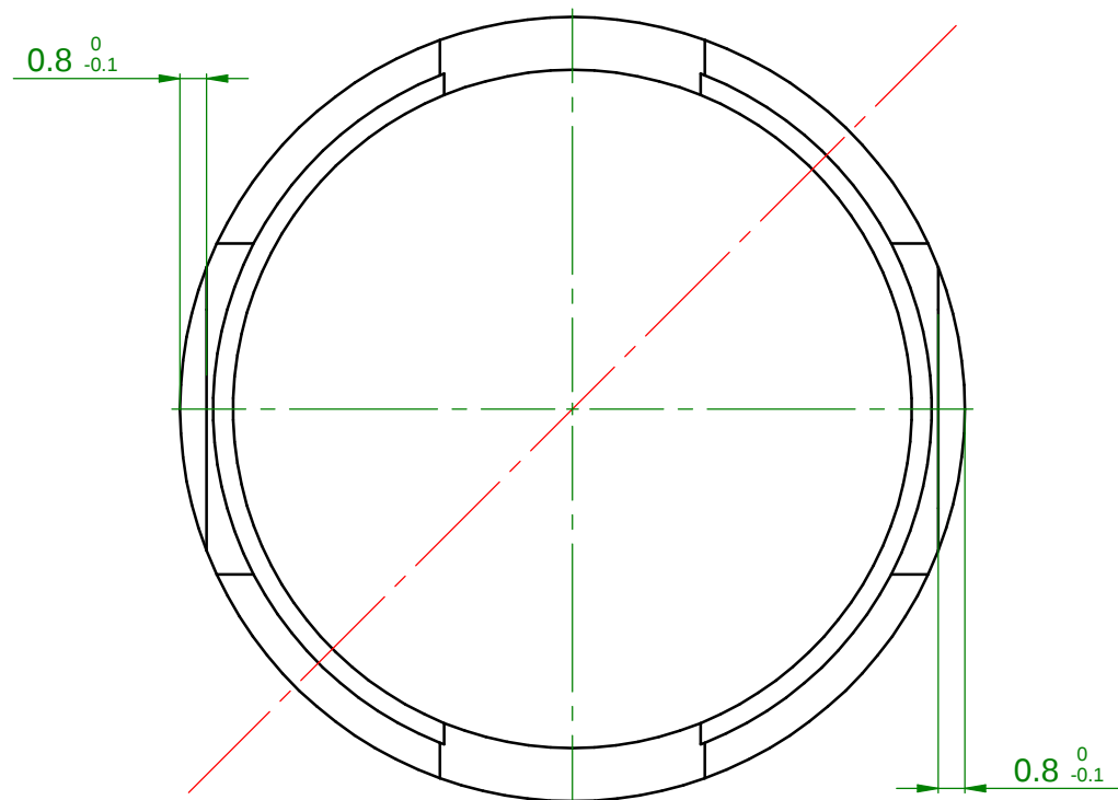
DETTAGLIO C
