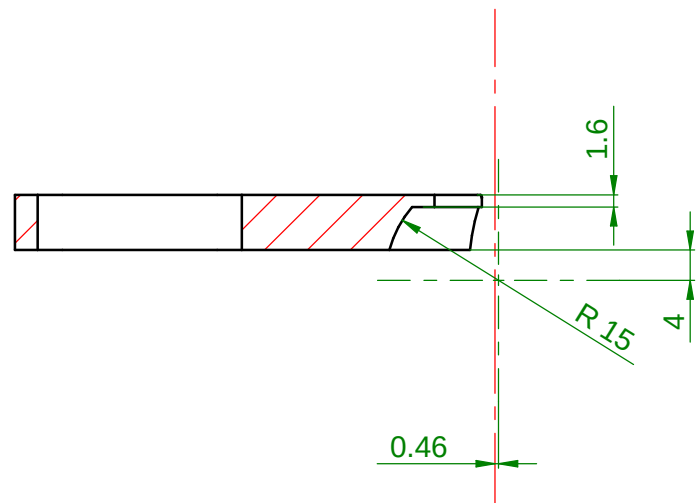
SEZIONE B-B
