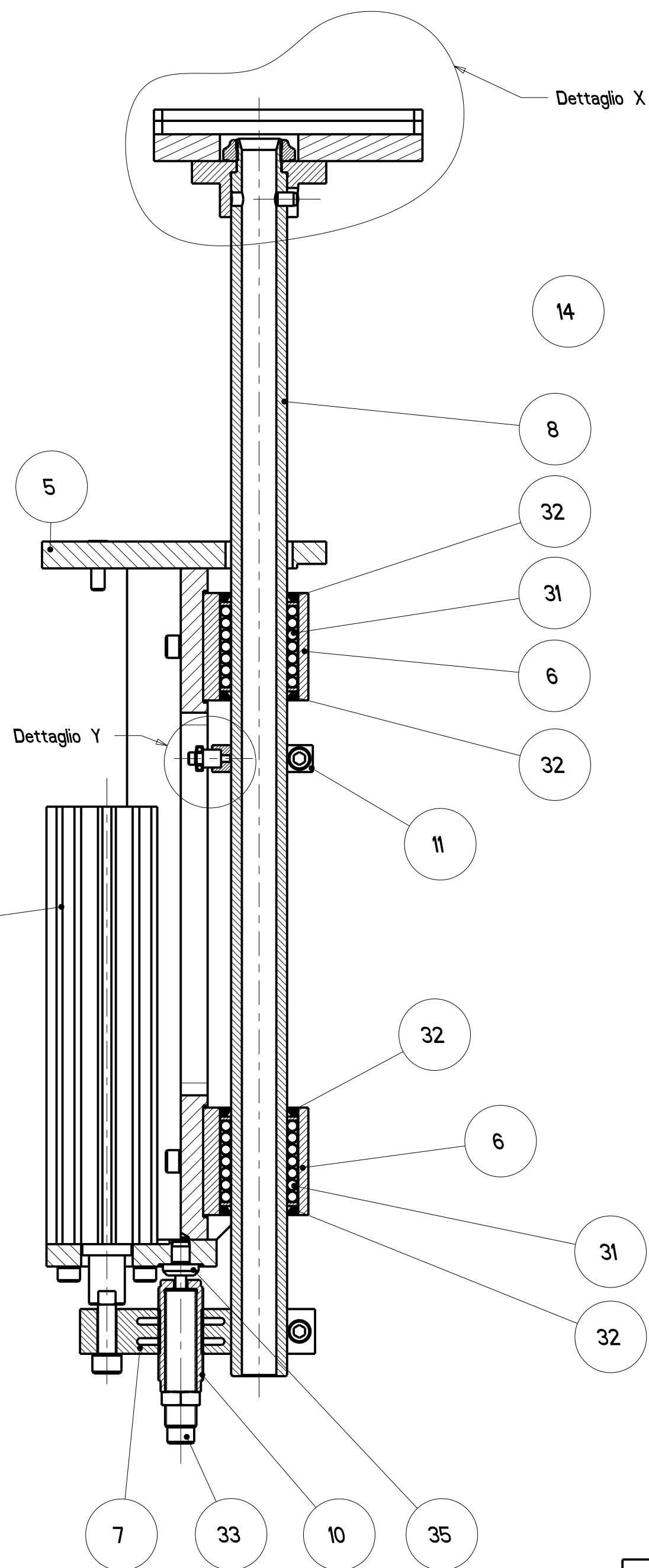
Sezione A-A
