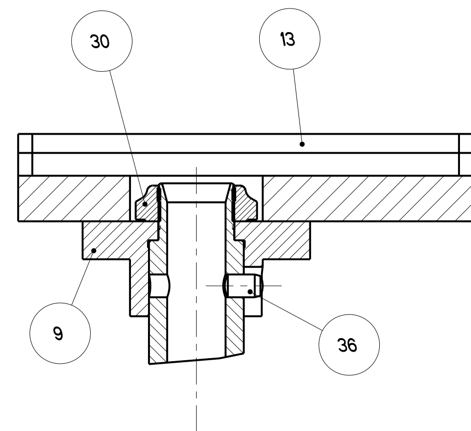
Dettaglio X Scala 1:1
