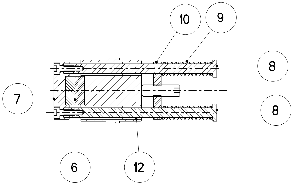
SEZIONE B-B
