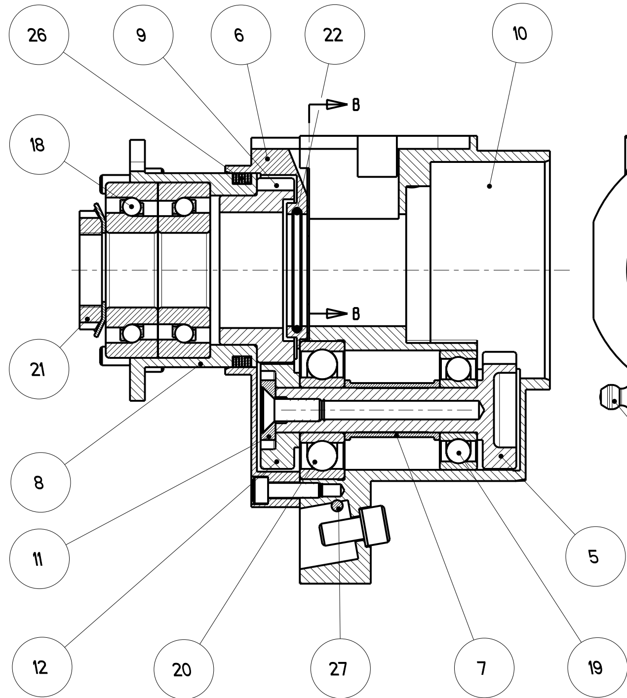
Sezione A-A
