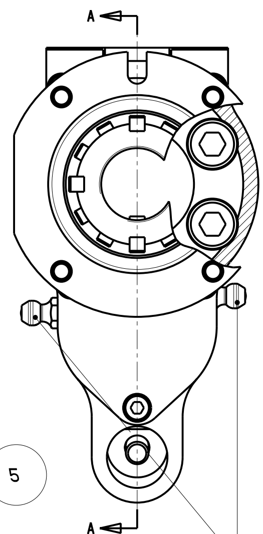
Sezione B-B
