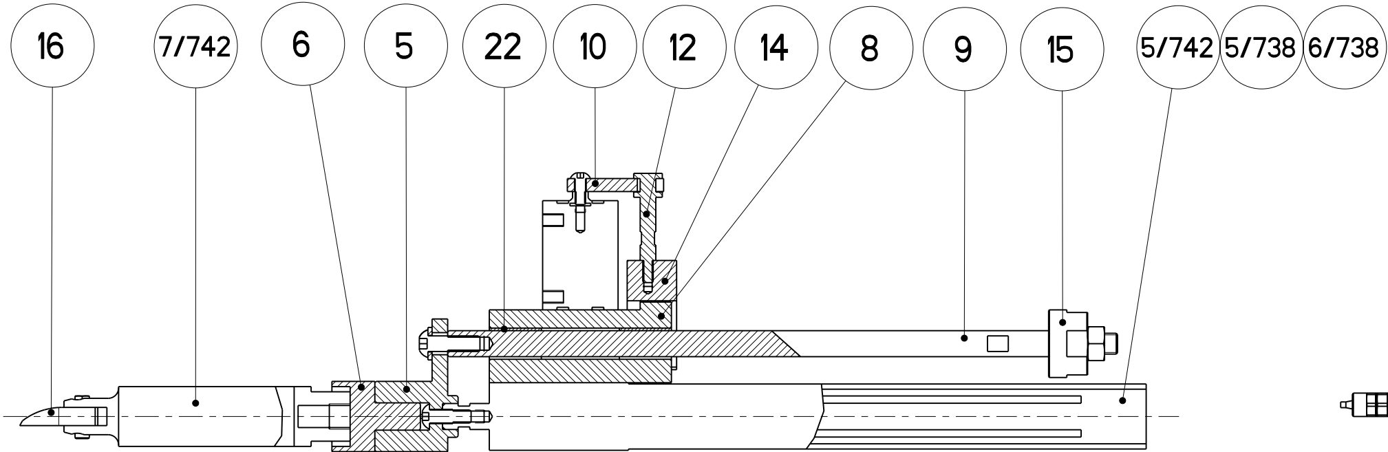
SEZIONE A - A
