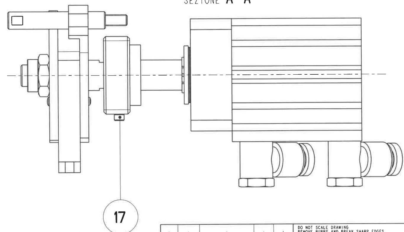
SEZIONE A-A
