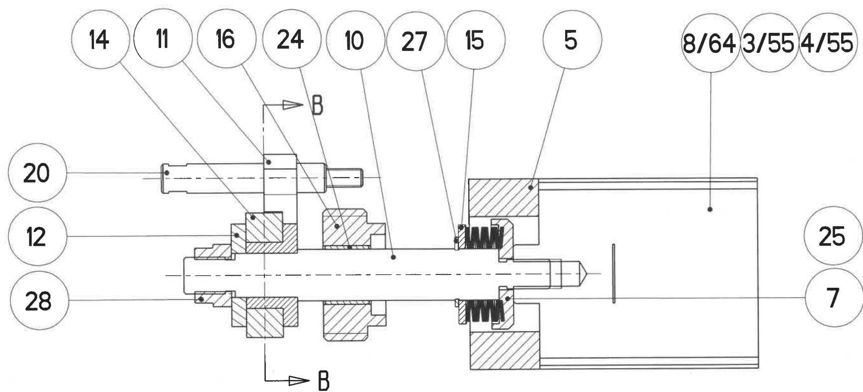
SEZIONE A-A
