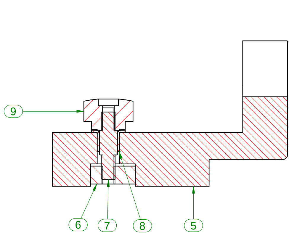
SEZIONE A-A
