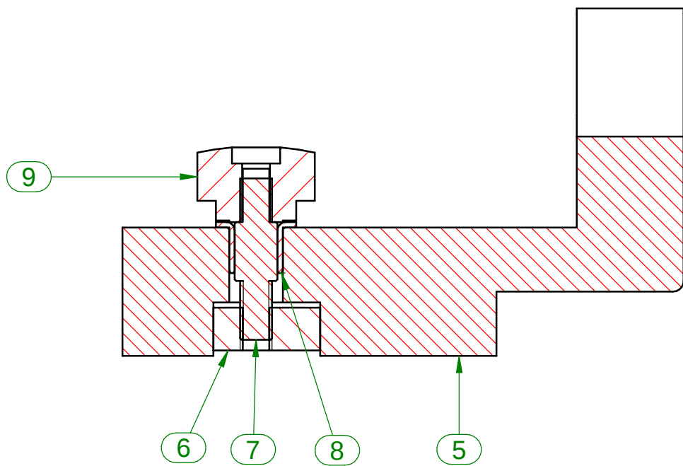
SEZIONE A-A
