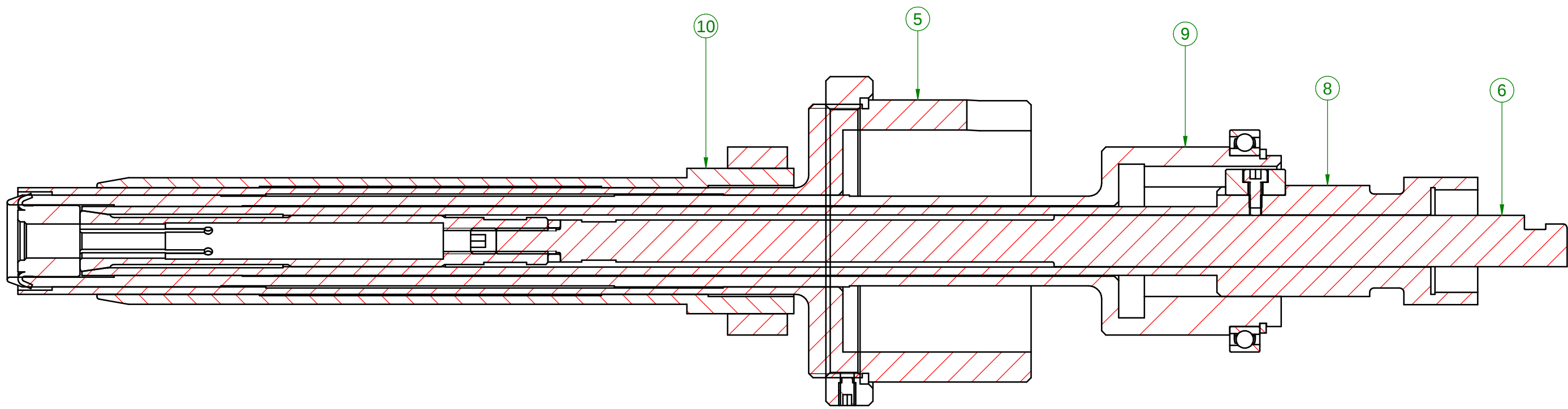
SEZIONE D-D
