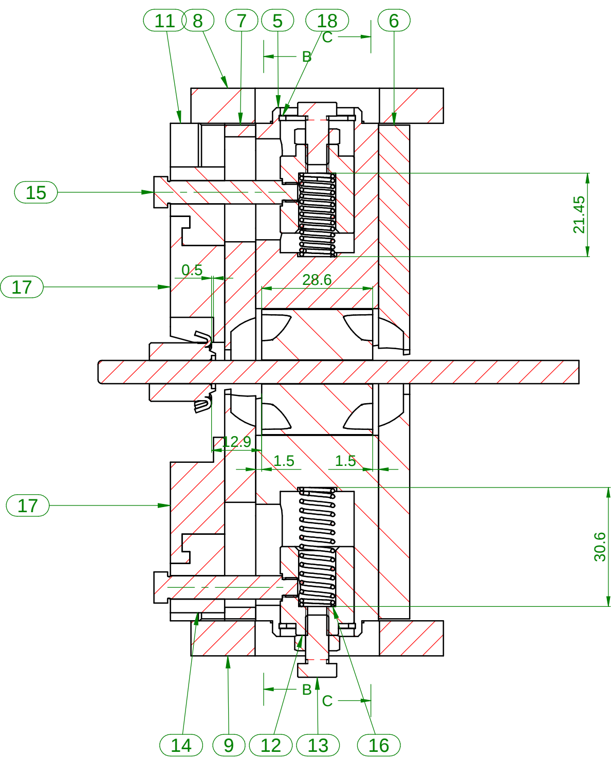
SEZIONE A-A
