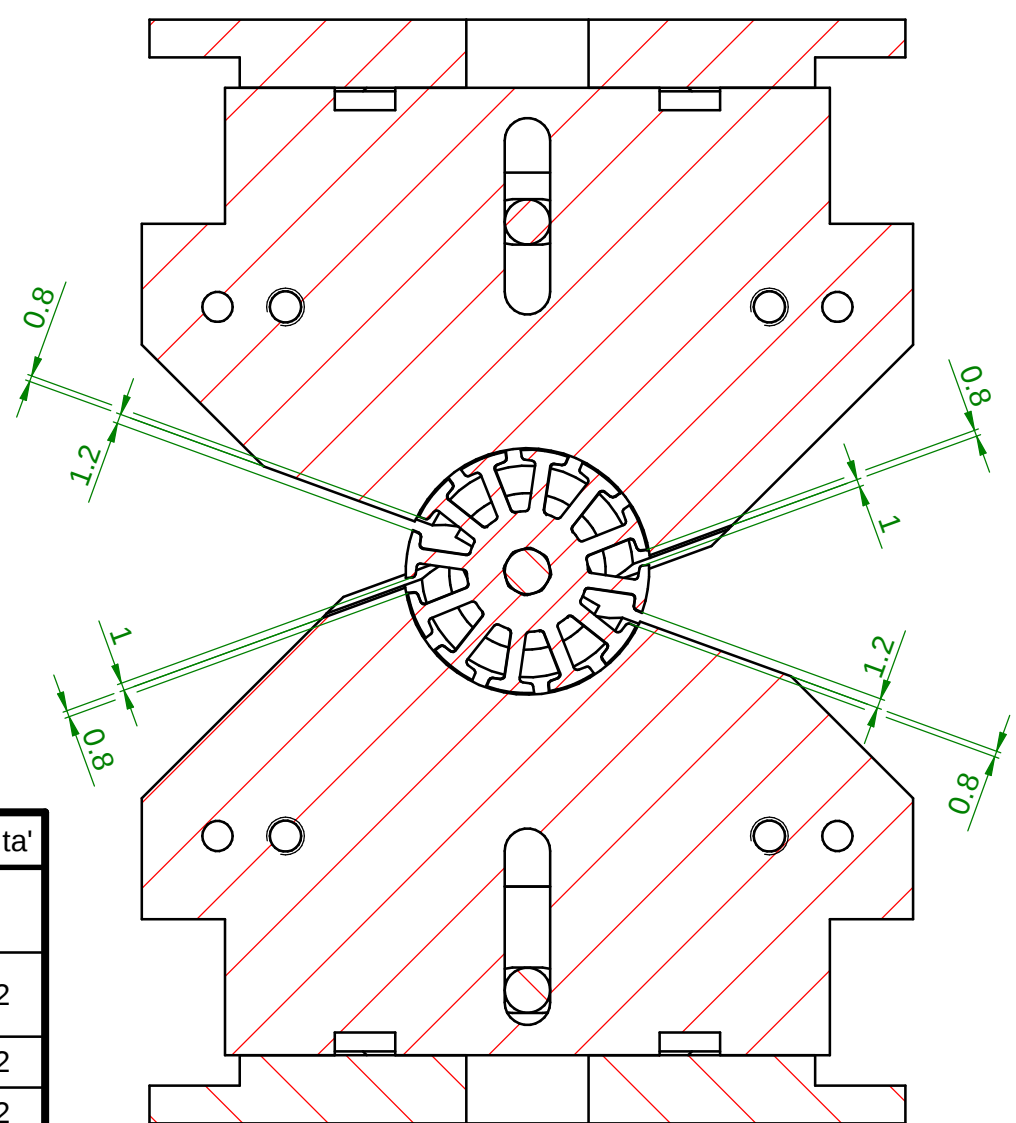
SEZIONE B-B
