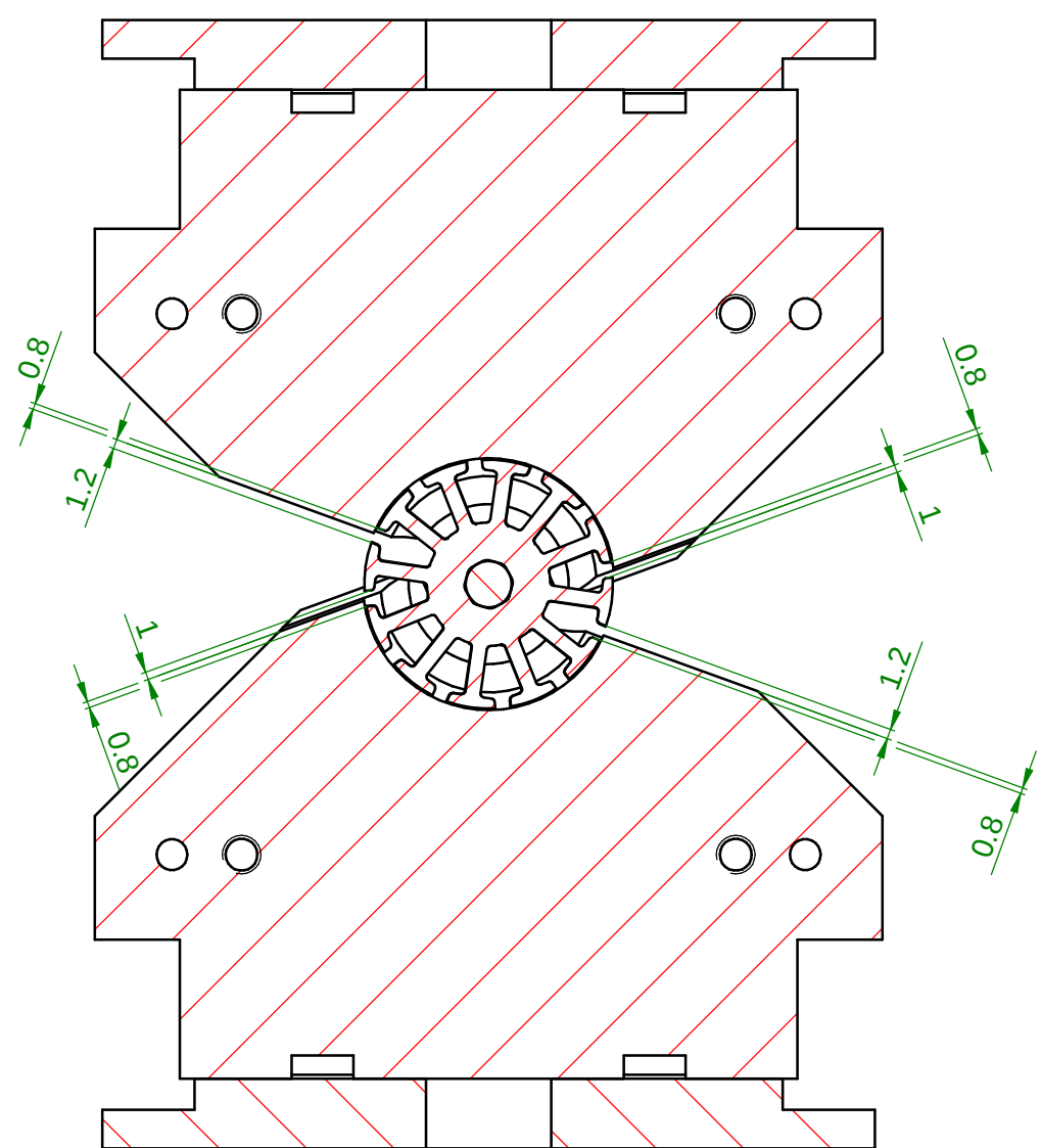
SEZIONE C-C
