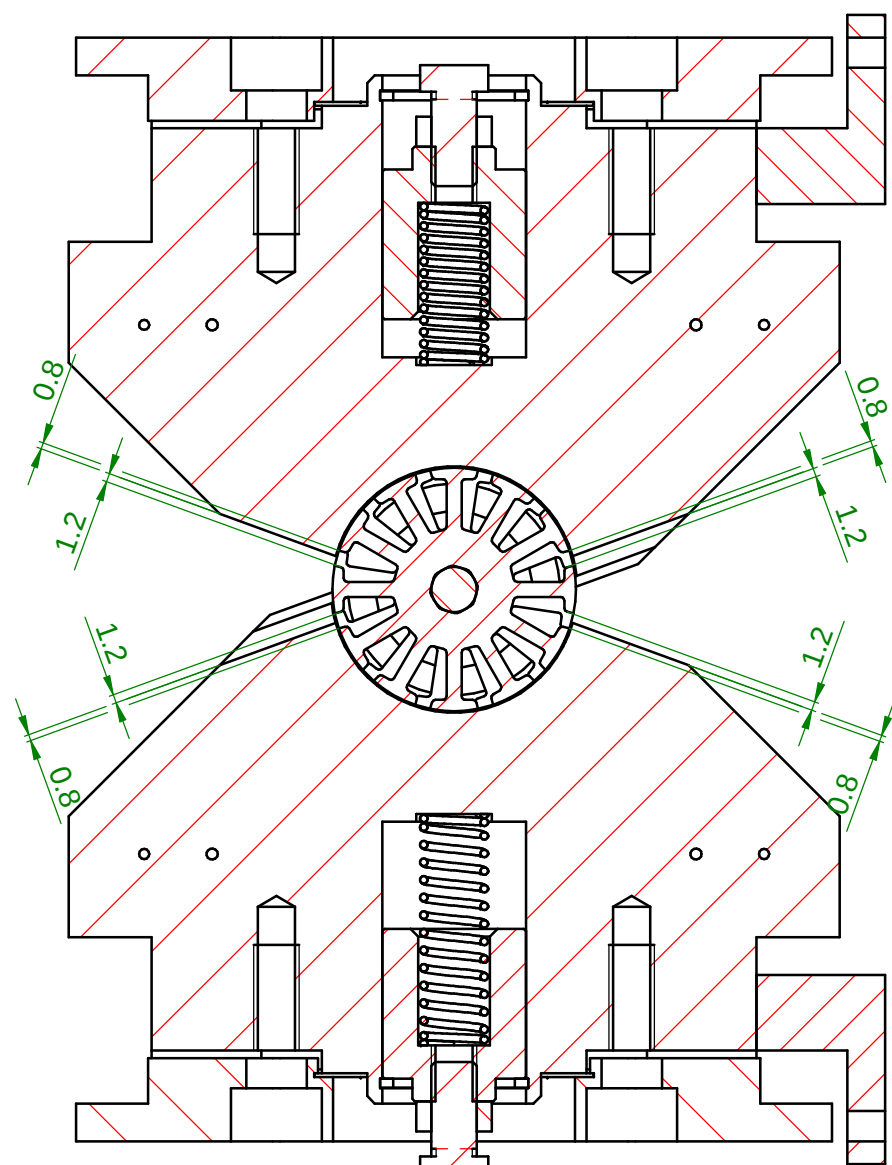
SEZIONE D-D
