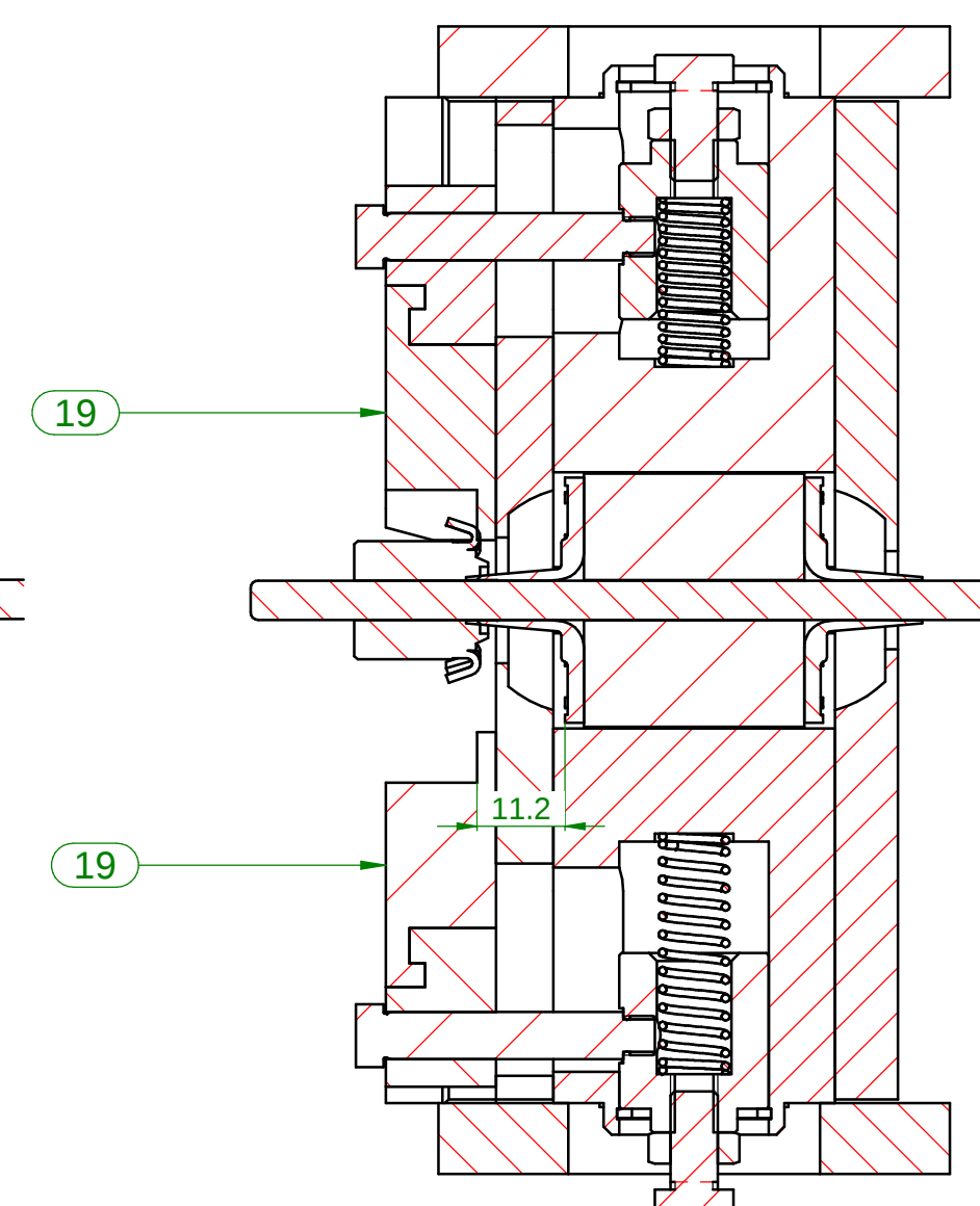
SEZIONE C-C
