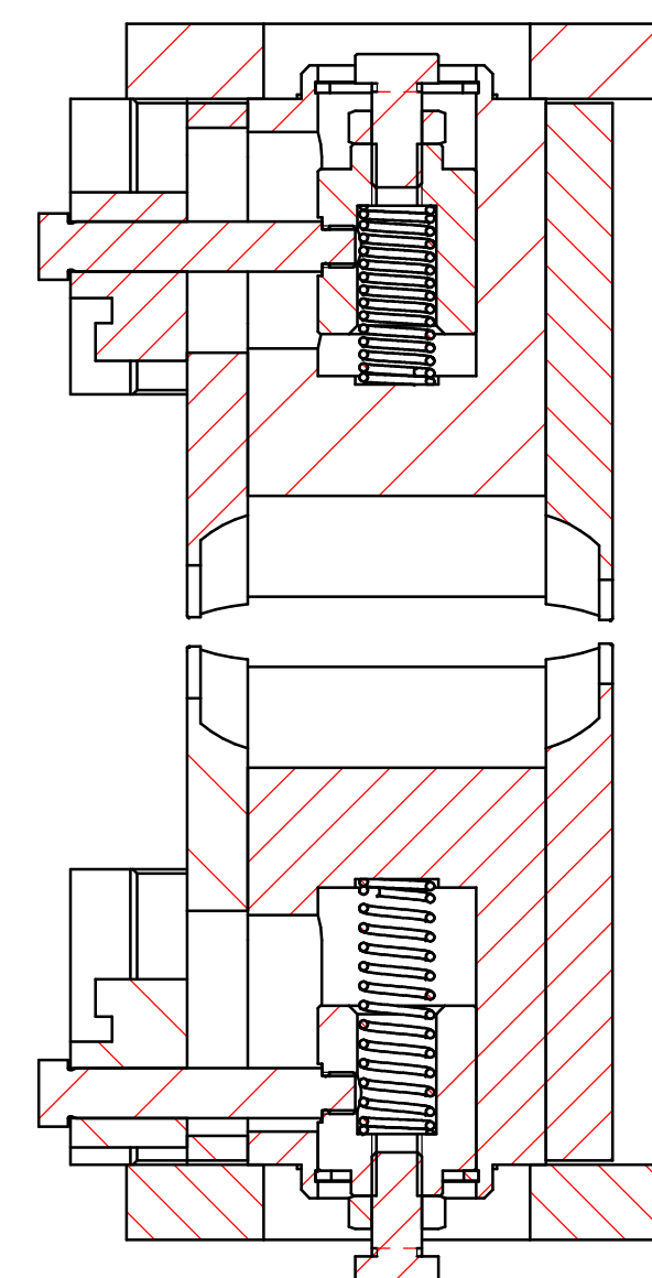
SEZIONE D-D
