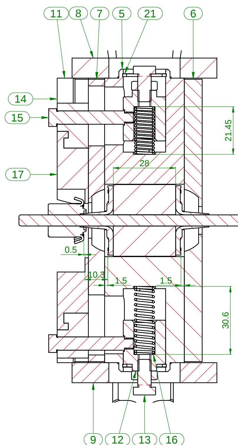
SEZIONE A-A
