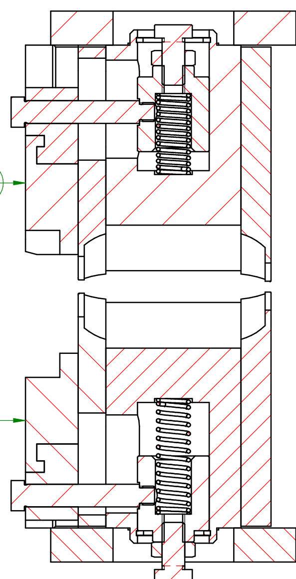
SEZIONE E-E
