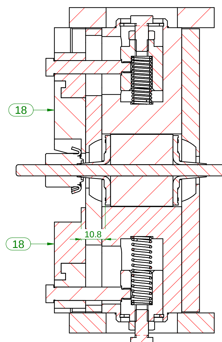
SEZIONE B-B
