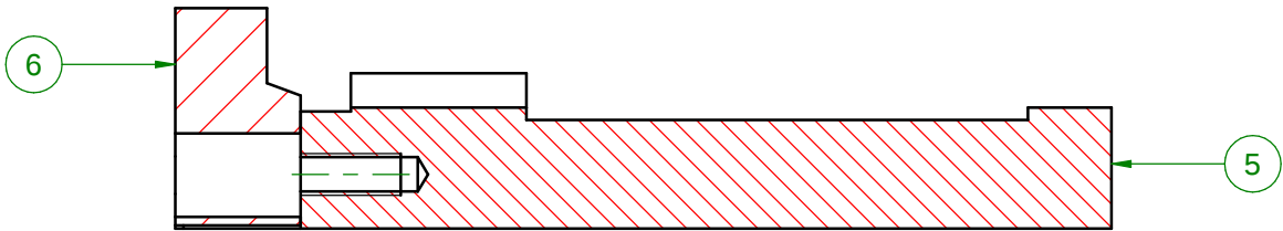
SEZIONE A-A
