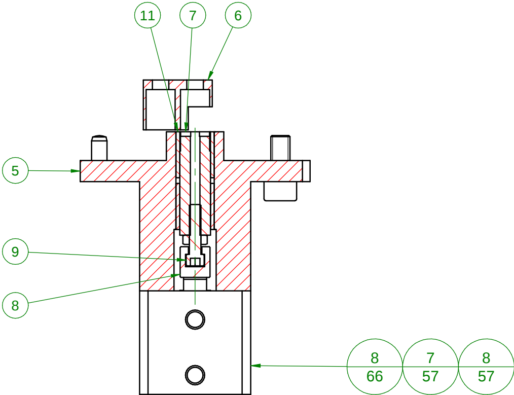
SEZIONE A-A
