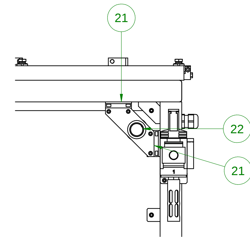
Vista parziale (senza pannello)
