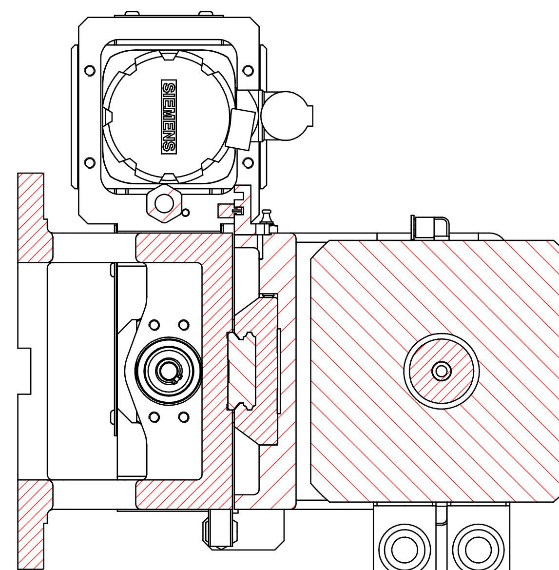
SEZIONE B-B
