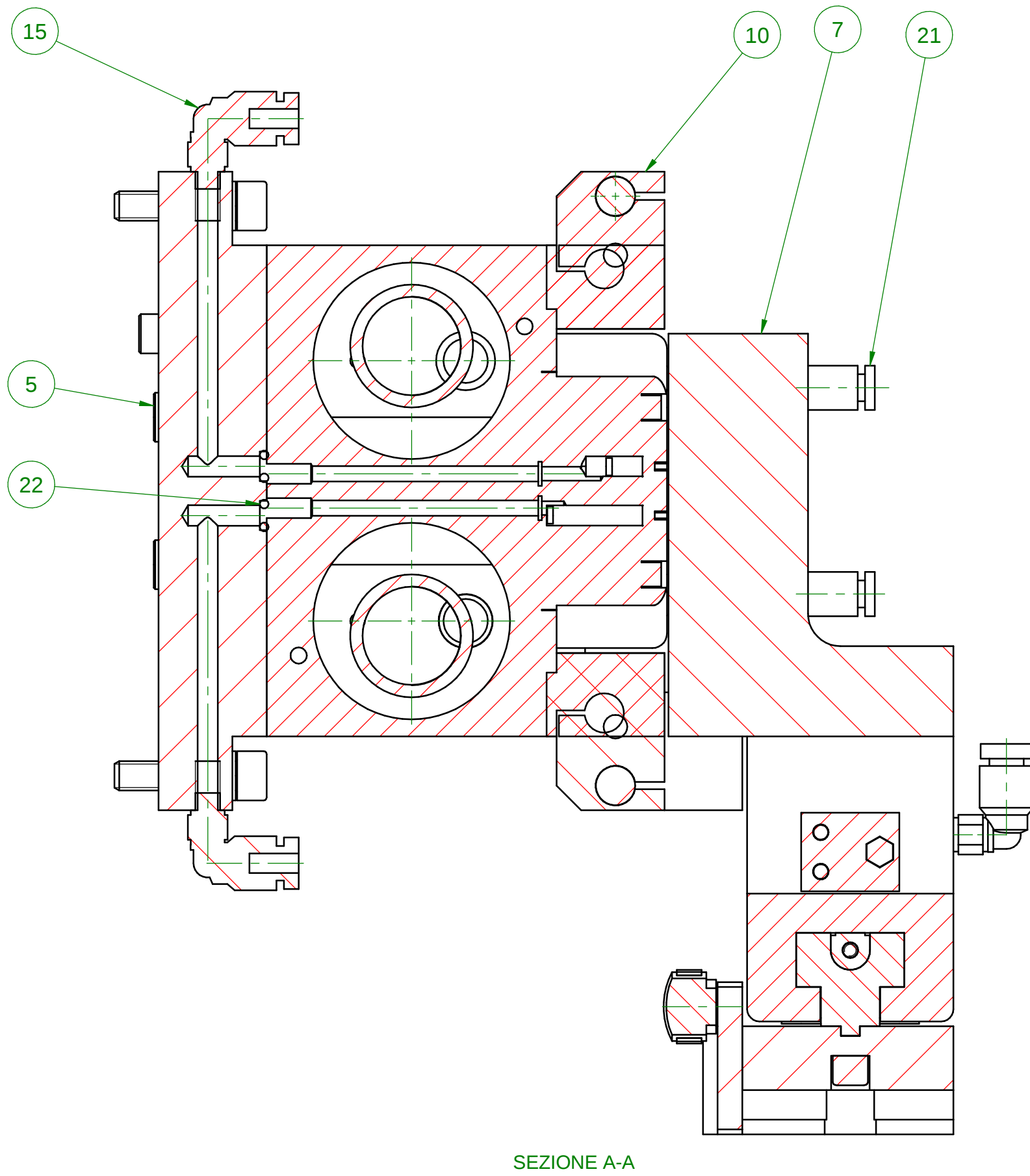
SEZIONE A-A
